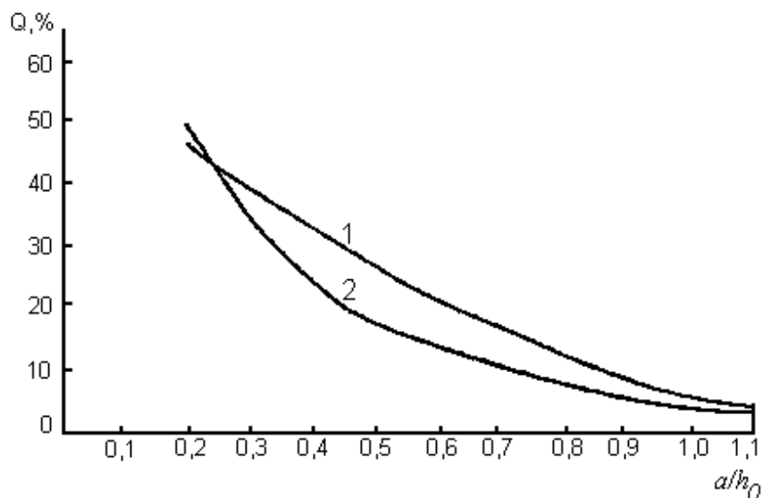
Рис.ПЗ.3. Зависимость доли перелившейся через обвалование жидкости
