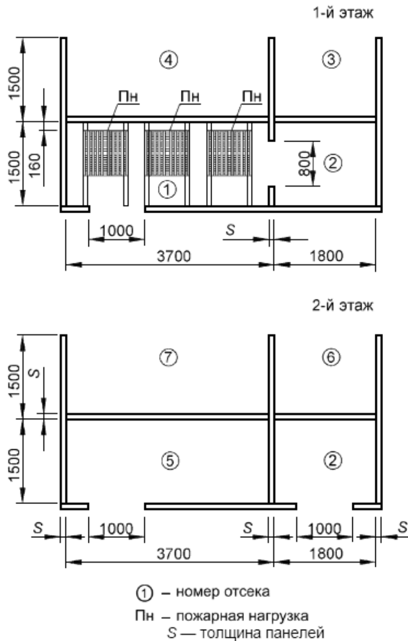
Рисунок Г.4 - Поэтажные планы
