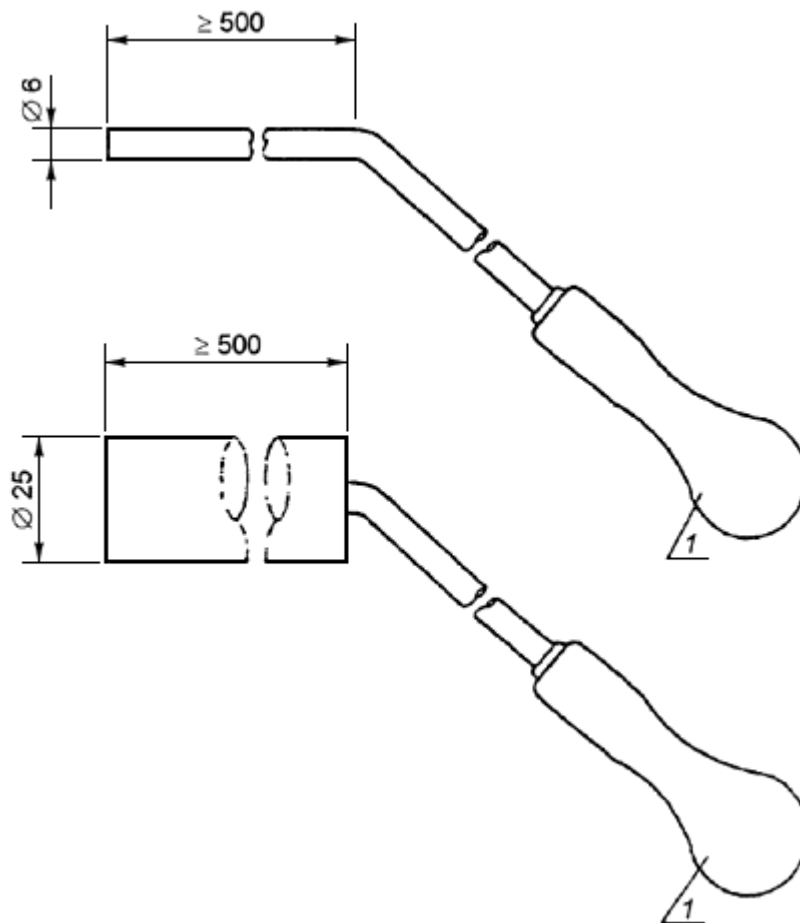
Рисунок А.1 - Конструкция щупов
