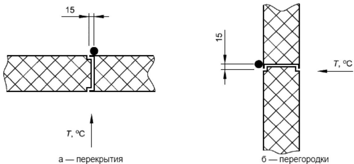
Рисунок Б.4 - Места установки термопар на стыках
