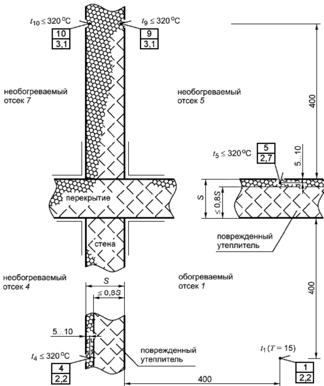
Рисунок Д.1 - Температуры в контрольных точках 4, 5, 9, 10 и повреждения панелей в месте пересечения стены и перекрытия между отсеками 1, 4, 5, 7
