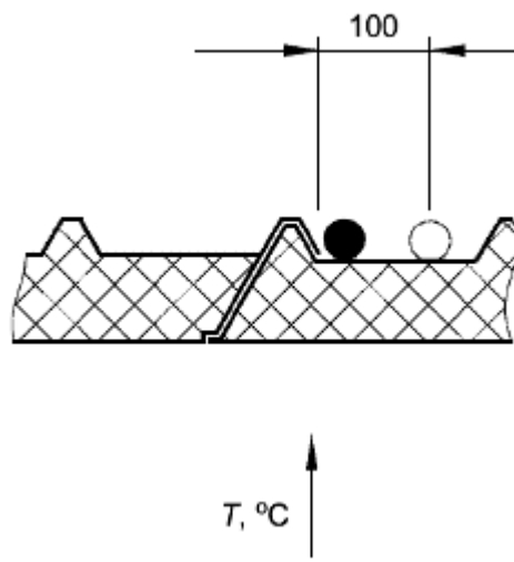
Рисунок Б.5 - Места установки термопар на гофрах покрытия
