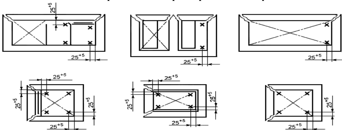
Рисунок Д.1 - Схемы расстановки термопар в объеме сейфа Приложение Е (рекомендуемое)
